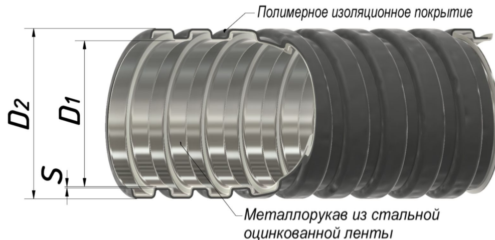
Рисунок 1. Шланг электромонтажный ШЭМ
