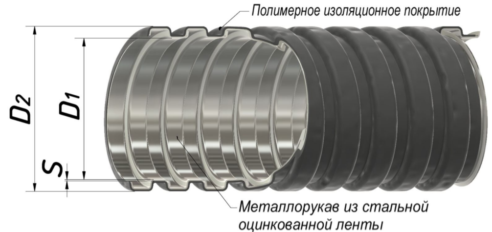
Рисунок 1. Металлорукав типа МРПИ нг морозостойкий
