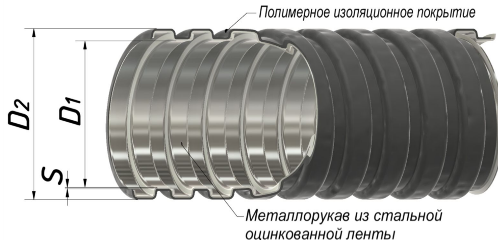
Рисунок 1. Металлорукав типа РЗ-ЦП нг с протяжкой
