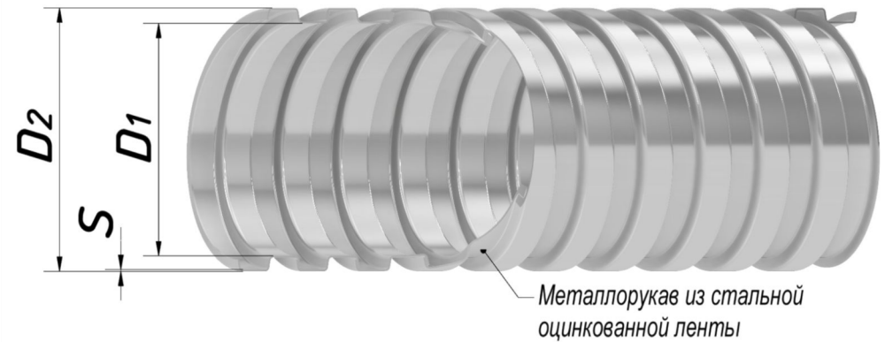
Рисунок 1. Металлорукав типа P3-Ц
