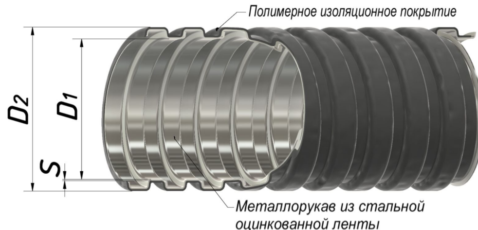
Рисунок 1. Металлорукав типа МРПИ нг морозостойкий с протяжкой
