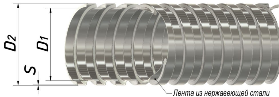
Рисунок 1. Металлорукав типа P3-N
