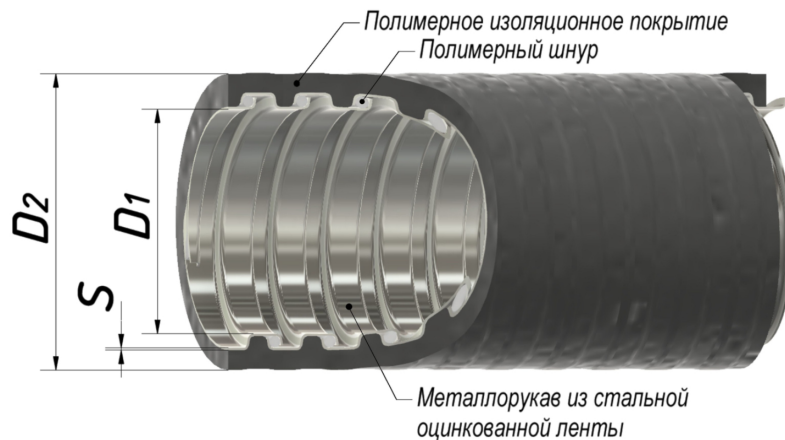
Рисунок 1. Металлорукав МПП нг HF черный
